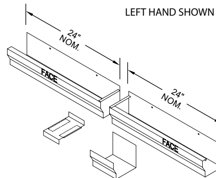
END CAP
