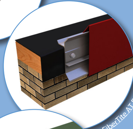
FiberTite 200 Fascia
